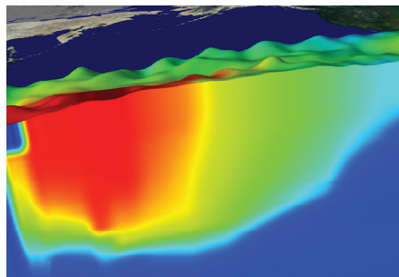
Fotografía de la portada: Durante el fenómeno meteorológico de El Niño. Vistas de la altura de la superficie del Océano Pacífico (representada por las olas en verde) y la temperatura del mar (representados por los colores). El color rojo representa 30° C hasta el azul que representa 8° C. La profundidad es hasta 200 m. Fuente: NASA/Goddard Space Flight Center Scientific Visualization Studio
